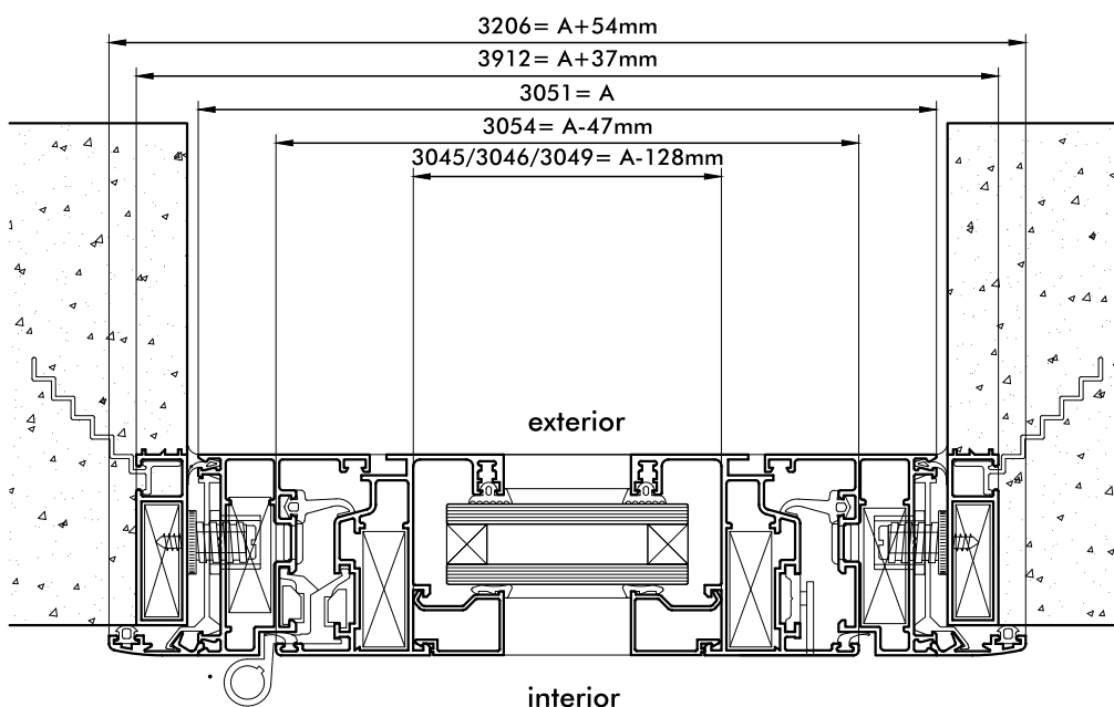
CORTE 1-2
