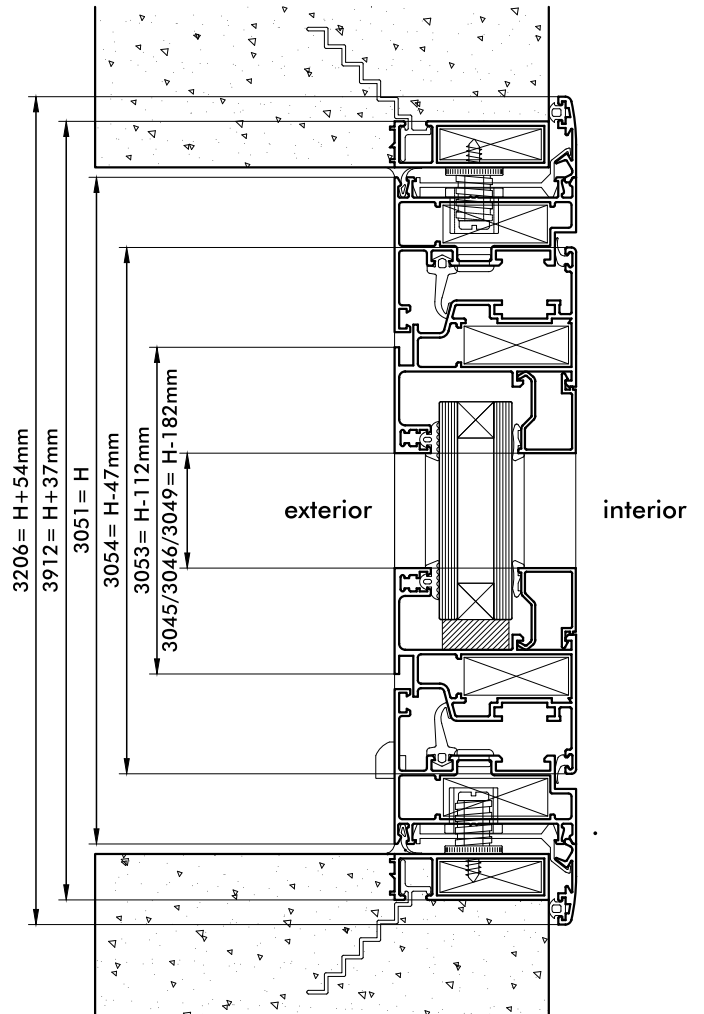
CORTE 3-4
