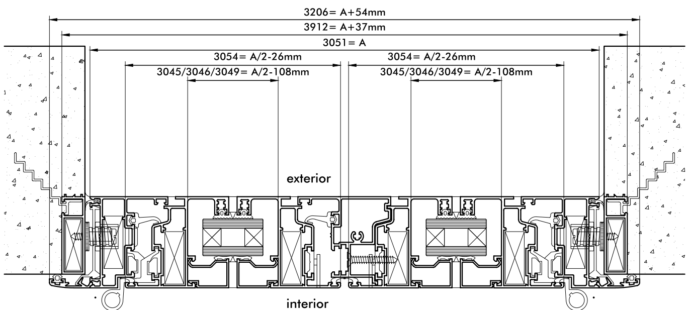
CORTE 1-2
